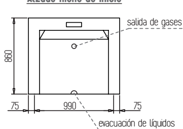
Alzado nicho de inicio
