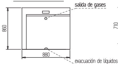
Alzado nicho central
