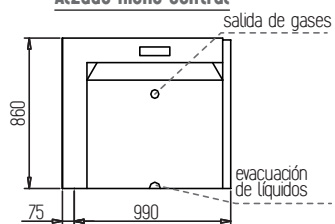
Alzado nicho central
