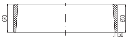
Sección longitudinal
